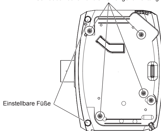
Die Positionen der Schraubenlöcher für die Aufhängevorrichtung und die einstellbaren Füße
